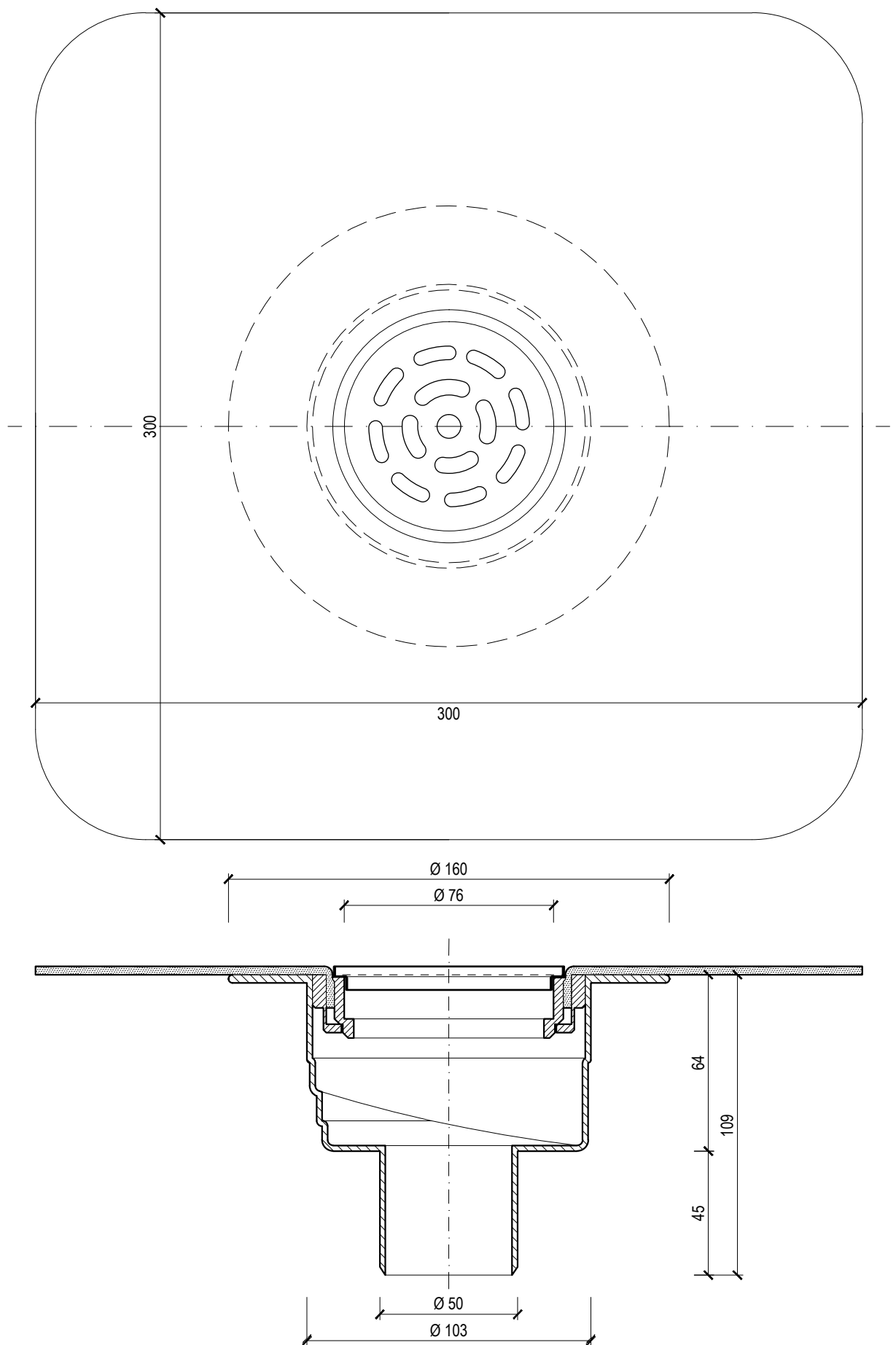
KF 6771 Flavent® Terrassen- / Dachablauf DN 50 senkrecht mit Bitumen-Manschette
