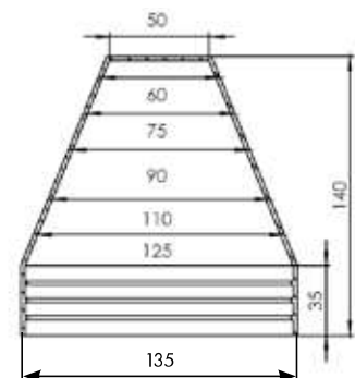
EPDM-Stufenmanschette für Flavent Dachdurchführungen DN 125
