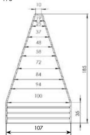
EPDM-Stufenmanschette für Flavent Dachdurchführungen DN 125
